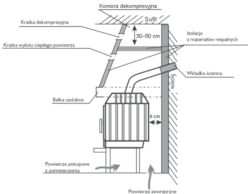
Rys. 4 Kominek – widok z boku
