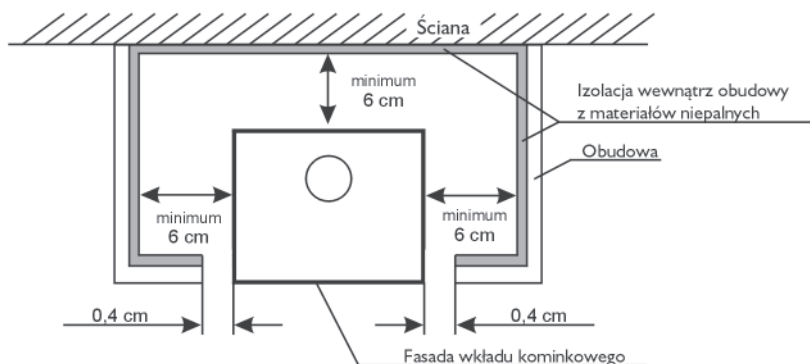
Rys. 3 Kominek – widok z góry
