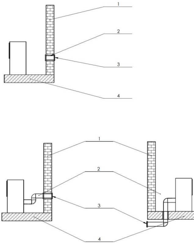
Rys. 3. [PL] Doprowadzenie powietrza/ [CZ] Přívod vzduchu/ [HU] Légbevezetés/ [SK] Prívod vzduchu/ [EN] Air supply/ [LT] Oro tiekimas/ [LV] Gaisa padeve/ [RU] Подача воздуха/ [EE] Õhuvarusustus/ [GR] Παροχή αέρα/ [RO] Alimentarea cu aer/ [BG] Подаване на въздух/ [UA] Подача повітря/ [NL] Luchttoevoer/ [HR] Dovod zraka/ [TR] Havanın beslenmesi/ [PT] Aporte de ar/ [FR] Arrivée d'air/ [ES] Suministro de aire
