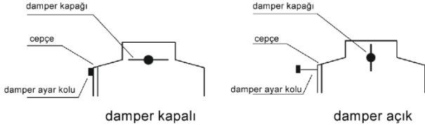
Şek. 5. Bir damper ayarı örneği
