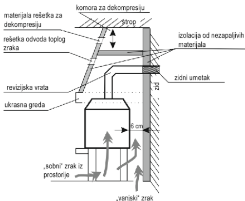
Crtež 3. Primjer načina ugradnje ugradbenih komina - floct i bokocrt
