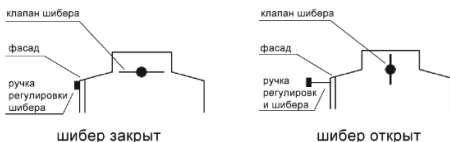
Рис. 5. Примерная регулировка шибера
