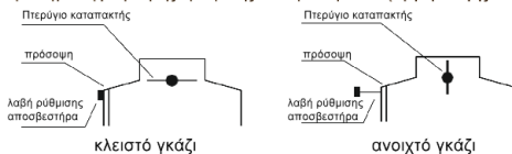
Σχ. 4. Παραδειγματική ρύθμιση της πρόσβασης του αέρα στην εστία (όψη πρόσοψης του τειφροδόχου)
