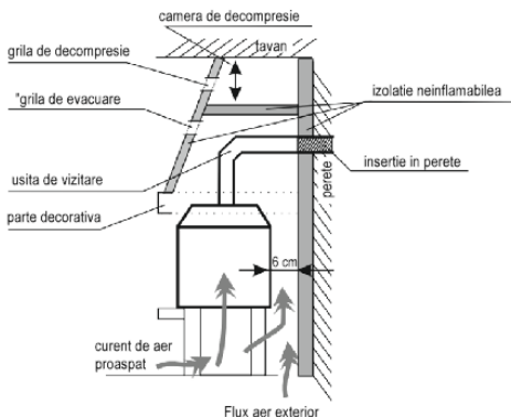
Fig. 3. Exemplu de instalare a unei insertii de semineu-vedere laterala
