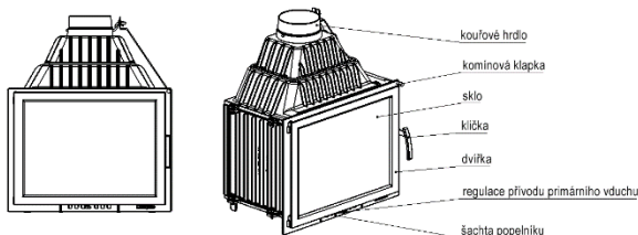
Obr. 1. Schéma křbové vložky
