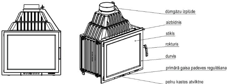
Att. 1 Kamīna ieliktna shēma.
