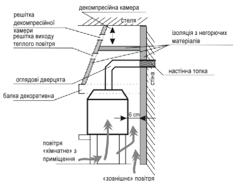
Рис. 3. Приклад способу установки камінної топки – вид зверху і збоку
