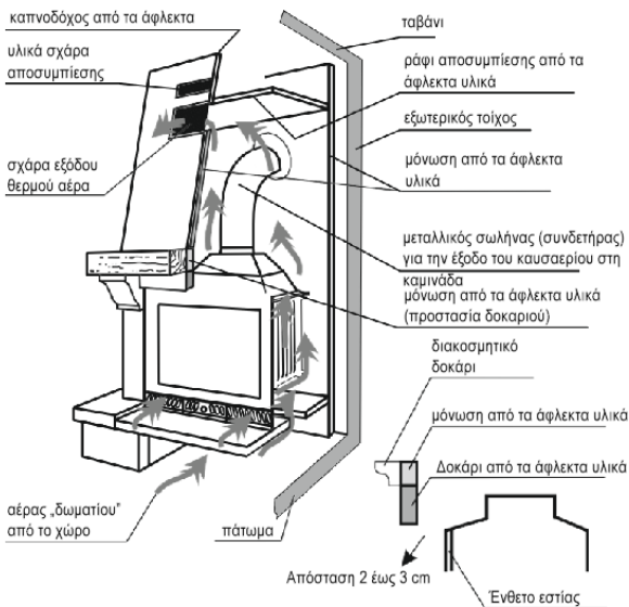
Σχήμα. 2. Παραδειγματικός τρόπος εγκατάστασης των ενθέτων τζακιών
