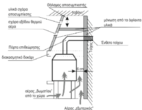
Σχ. 3. Παραδειγματικός τρόπος εγκατάστασης των ενθέτων τζακιών – όψη από πάνω και
