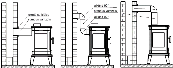
3 pav. Židininės krosnelės prijungimo schema
