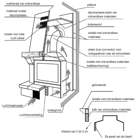
Afb. 2. Een voorbeeld van de installatie van haardpatronen
