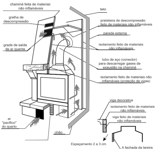
Figura 2. Exemplo de instalação da lareira.
