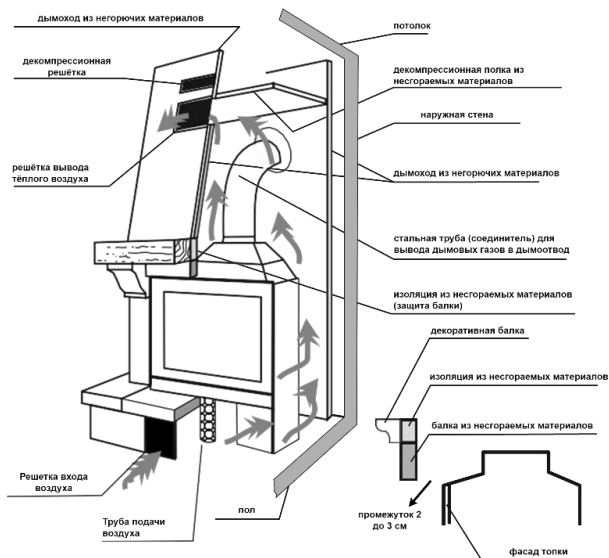
Рис. 2. Примерный способ инсталляции каминных вкладышей.
