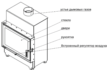
Рис. 1. Схема каминного вкладыша
