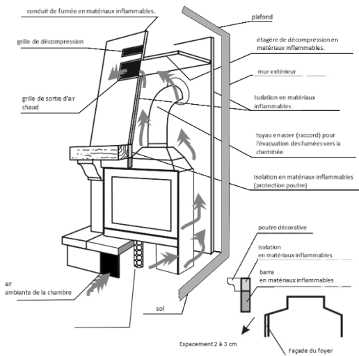
Fig. 2. Exemple d'installation d'inserts de cheminée
