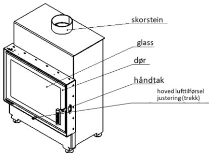
Figure 1 Skjema for peisinnsats
