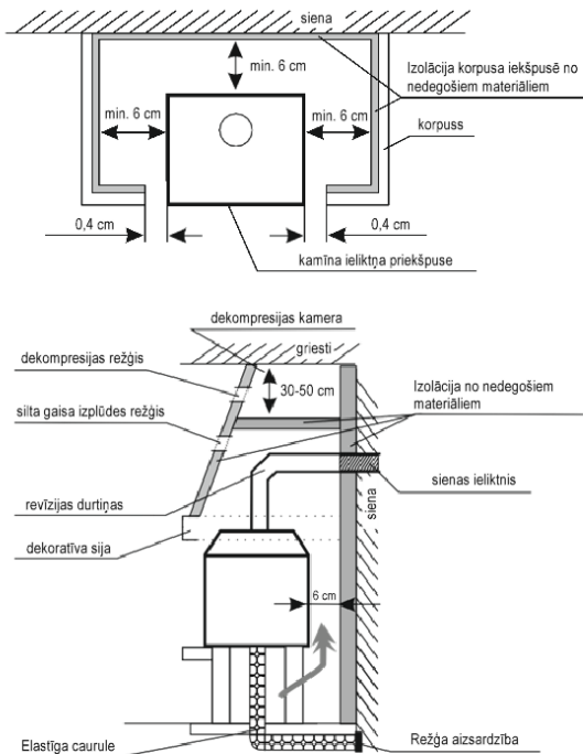
Att. 3 Piemērs, kā uzstādīt kamīna ieliktnus - skats no augšas un sāniem
