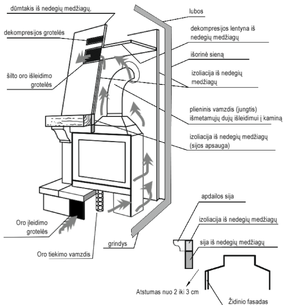
2 pav. Židinio įdėklų įrengimo pavyzdys
