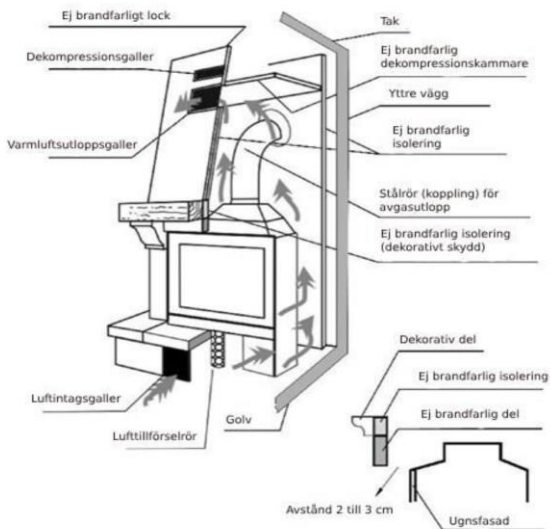
Figur 2. Ett exempel på hur man installerar eldstadsinsatserna
