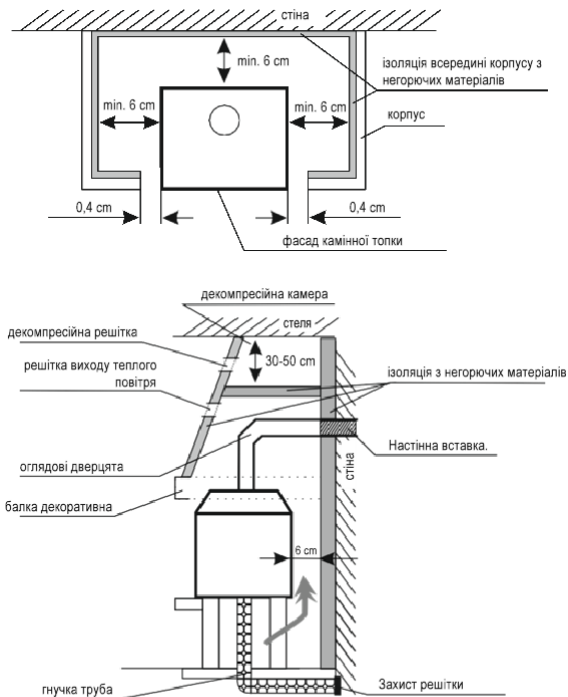
Рис.3. Приклад установки камінних топок - вид зверху і збоку.
