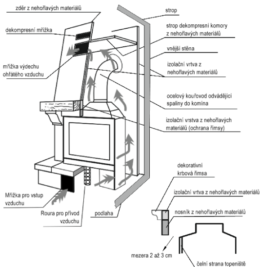
Obr. 2. Příklad montáže krbových vložek
