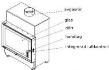
Figur 1. Schema för eldstadsinsats
