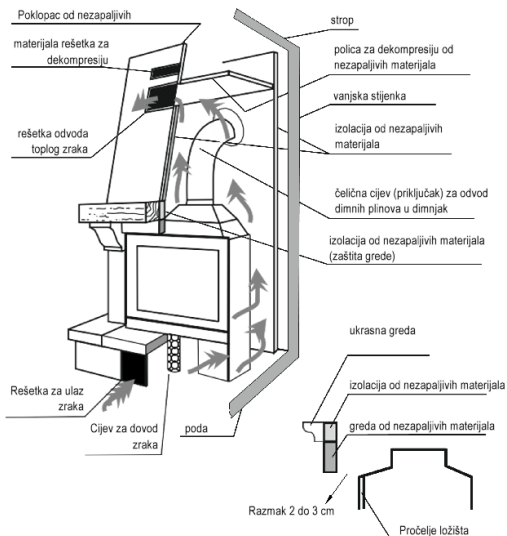
Crtež 2. Primjer načina ugradnje ugradbenih komina
