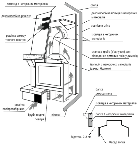
Рис. 2. Приклад способу установки камінної топки.
