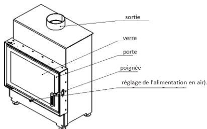
Fig. 1. Schéma de l'insert de cheminée.
