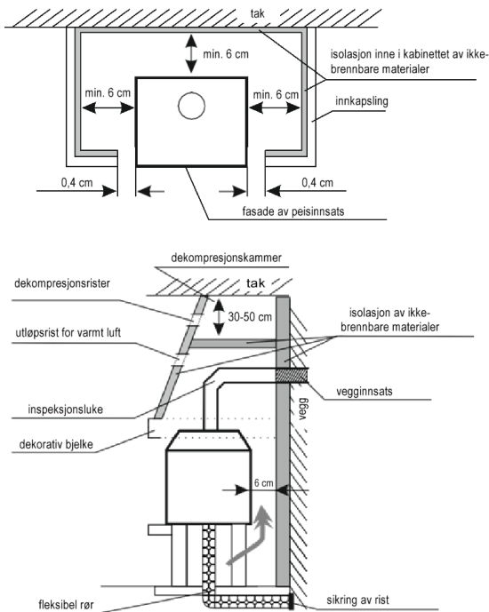
Fig. 2 Eksempel på montering av peisnnsats - topp og side
