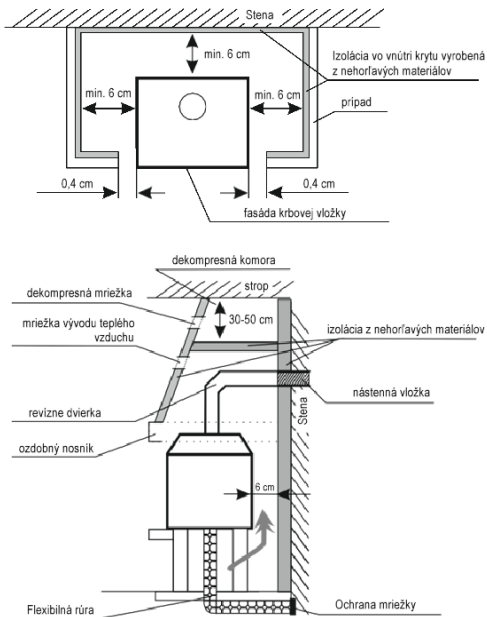
Obr. 3. Náznový spôsob inštalovania krbových vložiek - pohľad zhora a z boku
