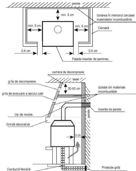
Fig.3. Un exemplu de instalare a unei insertii de șemineu - vedere de sus și laterală.
