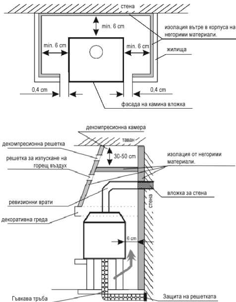
Фиг. 3. Пример за монтиране на камина за вграждане – горен и долен изглед
