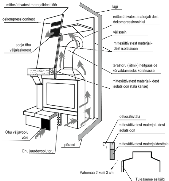
Joonis 2. Kaminasüdamiku paigaldusviisi näide.
