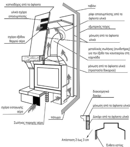
Σχήμα. 2. Παραδειγματικός τρόπος εγκατάστασης των ενθέτων τζακιών.
