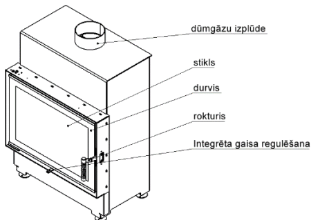
Att. 1 Kamīna ieliktna shēma
