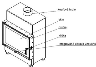
Obr. 1. Schéma krbové vložky.
