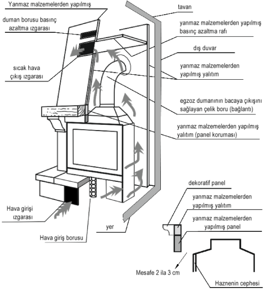
Şek. 2. Şömine haznelerinin kurulum şekli örneği
