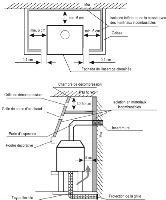
Fig. 3. Exemple d'installation d'inserts de cheminée - vue de dessus et de côté
