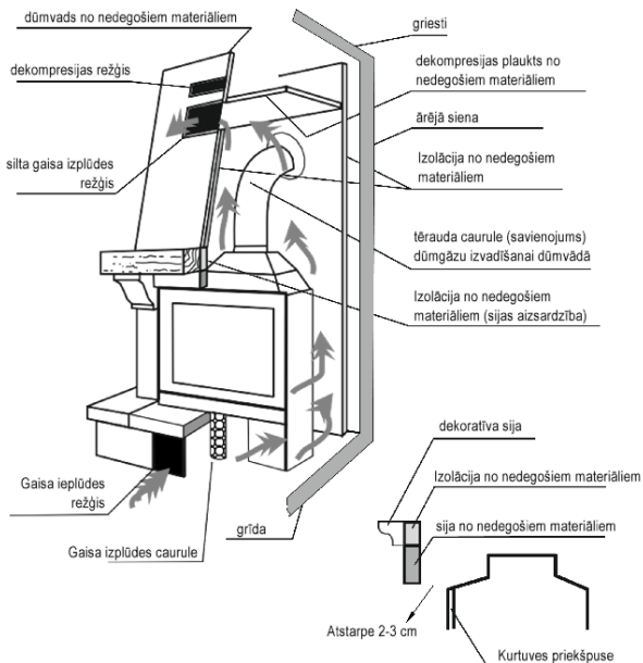
Att. 2 Piemērs, kā uzstādīt kamīna ieliktnis.
