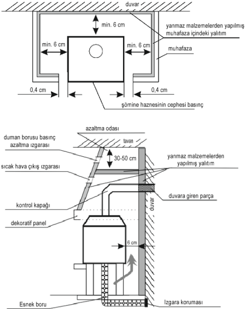
Şek. 3. Şömine haznelerinin kurulum şekli örneği - üstten ve yandan görünüm
