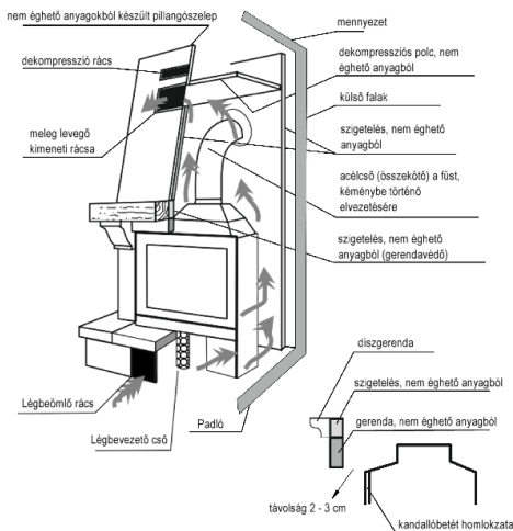
2 sz. Rajz. Példa a kandallóbetétek telepítésére.
