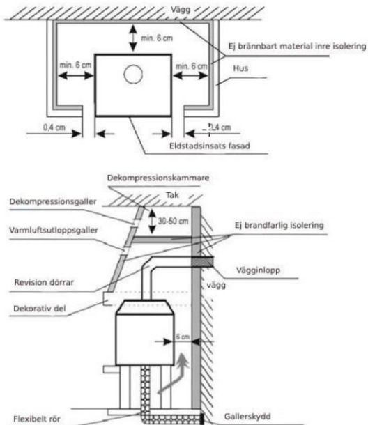
Figur 3. Exempel på installation av eldstadsinsatsen - topp och sida
