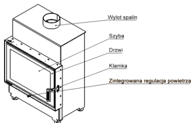
Rys. 1. Schemat wkładu kominkowego
