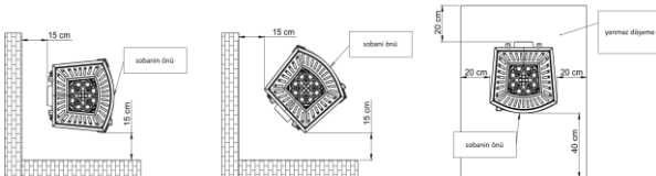
şek. 2. Ocağın yanıcı olmayan parçalara güvenli mesafeleri.
