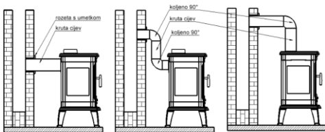
Crtež 3. Shematski prikaz priključivanja kaminske peći
