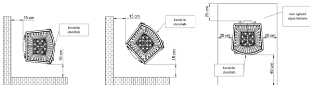
2 sz. Rajz. A kályha biztonságos távolsága a ne éghető részekről.
