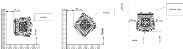
Joonis 2. Ahju ohutu kaugus mittesüttivatest osadest.
