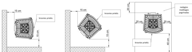
2 pav. Saugūs krosnies atstumai nuo nedegių dalių.
