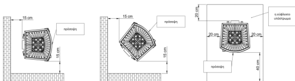
Ασφαλείς αποστάσεις θερμαντικού σώματος από μη εύφλεκτα μέρη.
