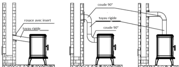
Fig.3. Schéma de raccordement du four de cheminée.
